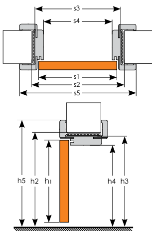
MODULINIŲ DURŲ BE UŽLAIDOS VARČIOS IR REGULIUOJAMOS STAKTOS MATMENYS (mm)
