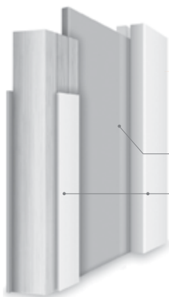
PAVYZDINIS VARČIOS SKERSPJŪVIS MODULINĖ D'ARTAGNAN
